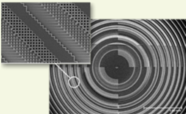
2 REM Aufnahme der CGH Nano-Struktur. | SEM image of the CGH's nano-structure.
