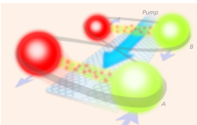
2 Schema eines periodischen Wellenleiters zur Erzeugung verschränkter Photonen durch zwei Konversionsprozesse A und B, die Signal- und Idlerphotonen jeweils in entgegengesetzte Propagationsrichtungen emittieren. |
