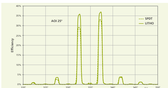
2 Beugungseffizienzmessung in TE- und TM-Polarisation für eine Inzidenz von 25^\circ bei \lambda = 532 \text{ nm} . | Diffraction efficiency measurement in s- and p-polarization for \lambda = 532 \text{ nm} and 25^\circ angle of incidence.
