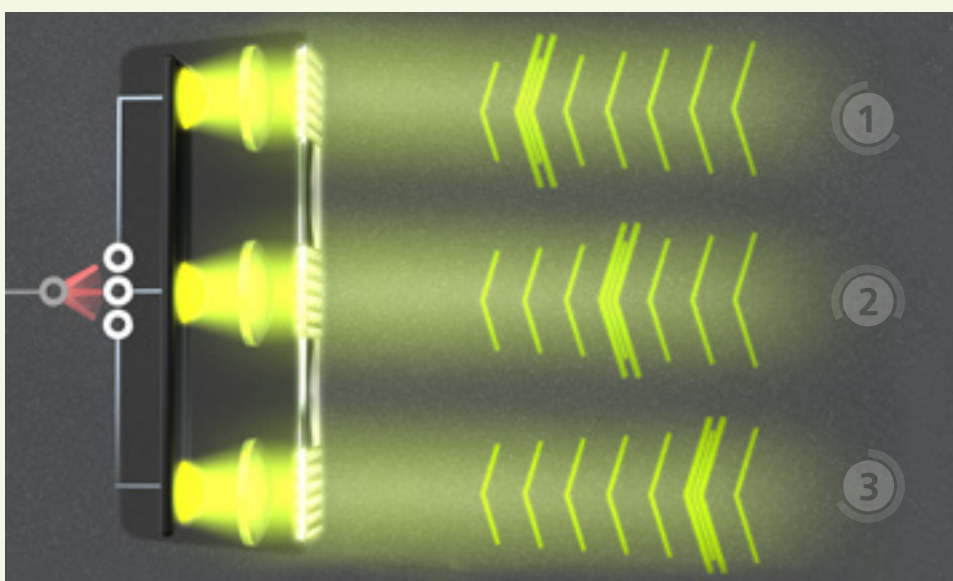
3 Optikschemata zur Projektion schaltbarer Bildinhalte. | Optics scheme for projection of switchable image content.
