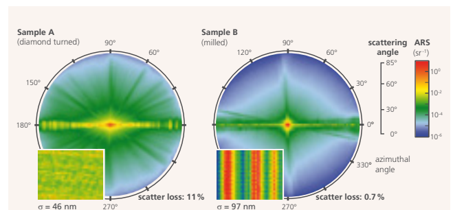
2 Hemisphärische Streulichtmessungen und Weißlichtinterferometermessungen an PMMA-Oberflächen für Beleuchtungsoptiken. | Hemispherical light scattering measurements and white light interferometer measurements on processed PMMA surfaces for imaging applications.
